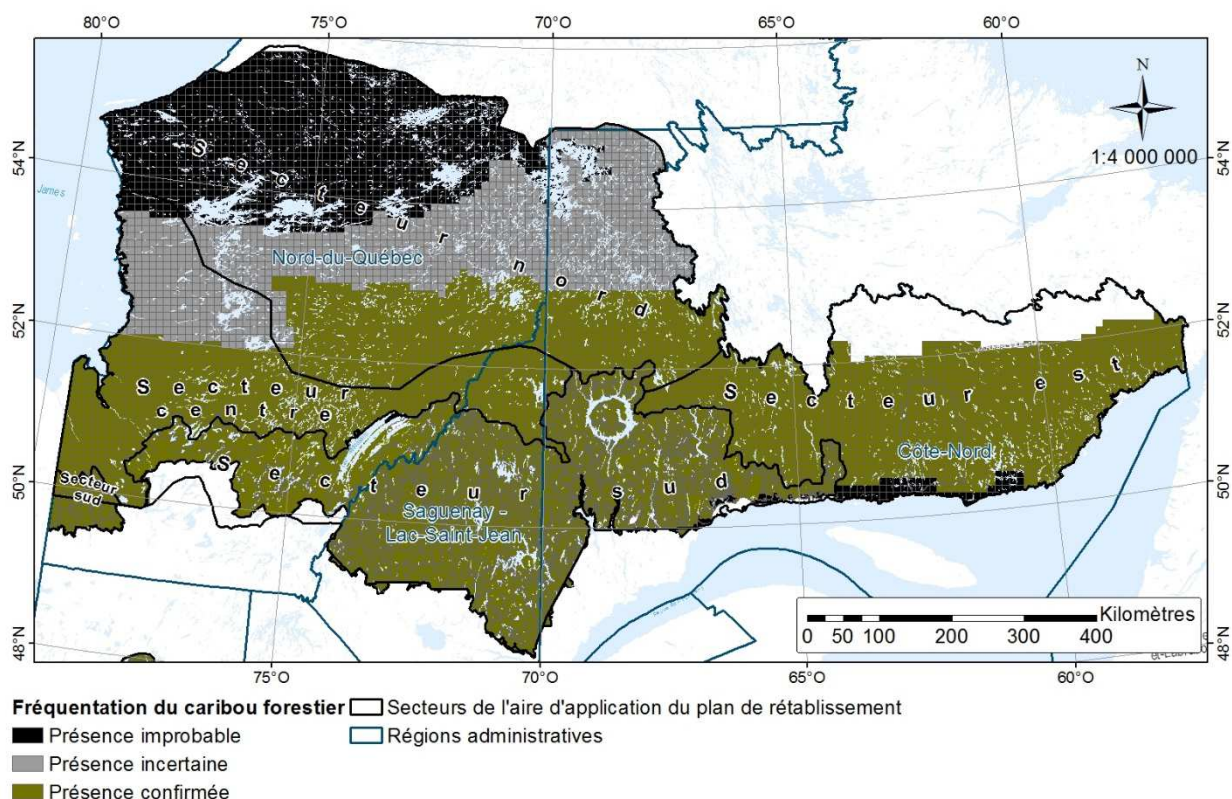
Figure 13. Fréquentation effective du caribou forestier d'après les observations et les connaissances pour les territoires les plus au nord et à l'est de l'aire d'application du Plan de rétablissement du caribou forestier.
