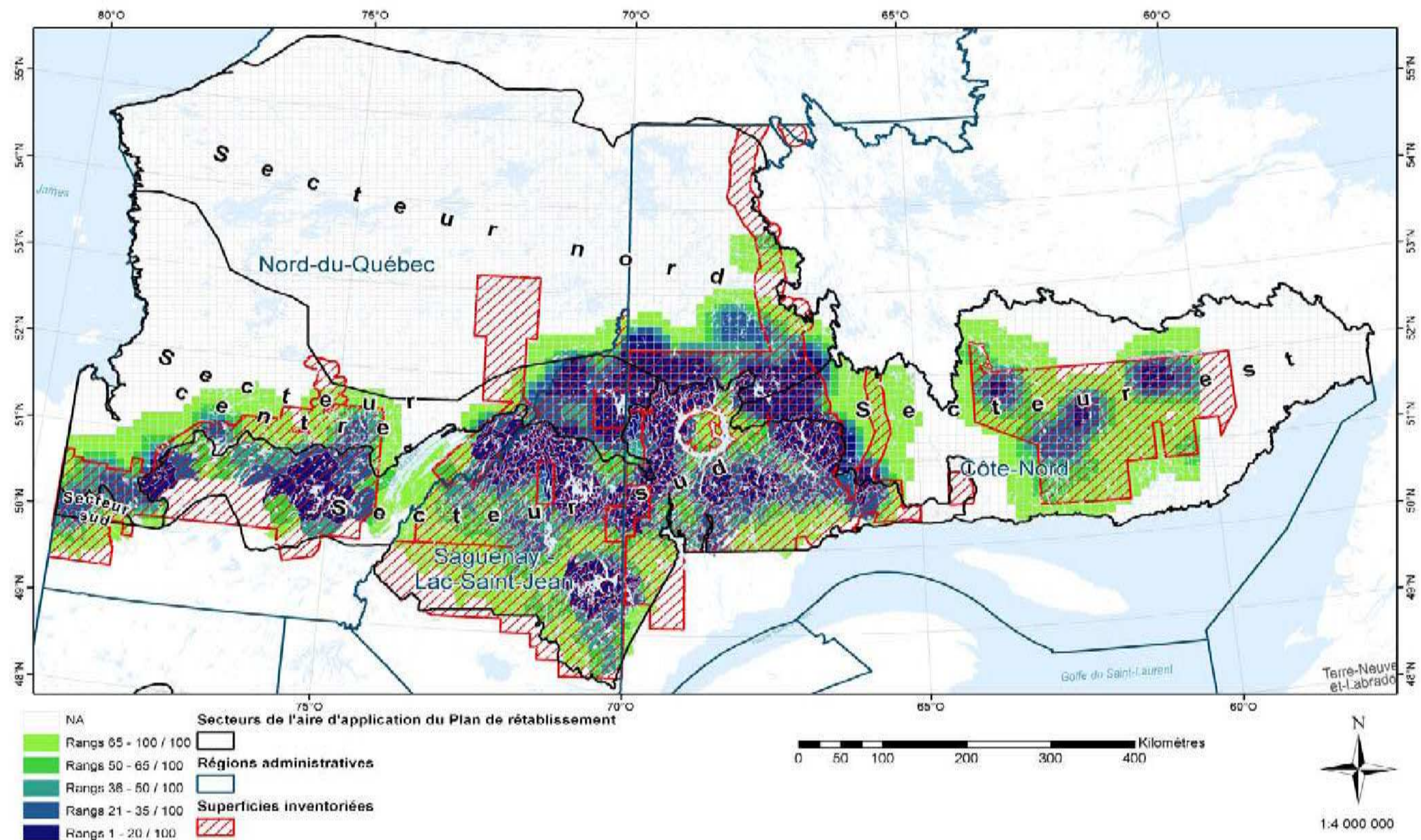
Figure A4.12. Variation spatiale dans les valeurs associées à l'analyse de la densité de noyaux de ravages de caribous forestiers issus des inventaires aériens, par COS ou UTR et superficies inventoriées de 1999 à 2014 ayant servi à l'analyse de la densité de noyaux.
