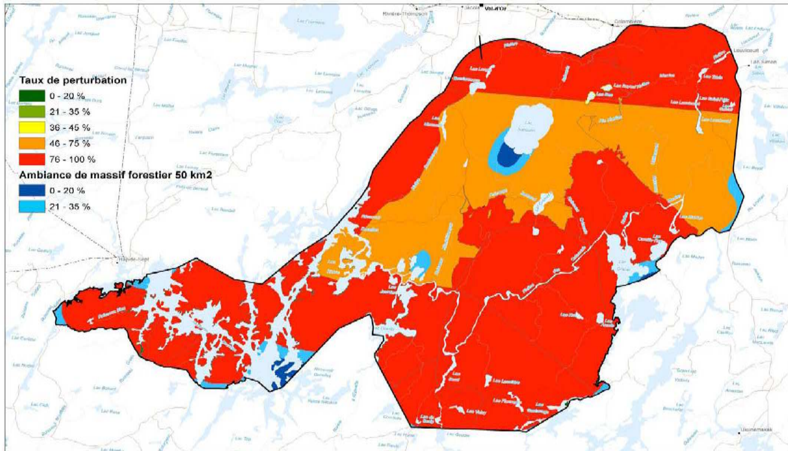
Figure A4.21. Taux de perturbation totale par COS/UTR et localisation des massifs forestiers résiduels dans le Plan d'aménagement du caribou de Val-d'Or à l'aide de l'ambiance de perturbation totale à 50 km².
