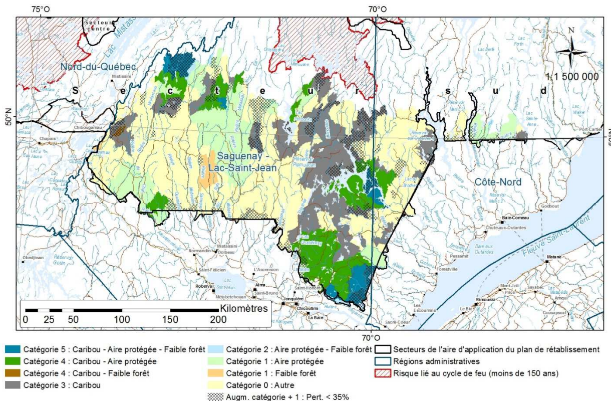
Figure 19. Caractérisation des paysages de perturbations permanentes par leurs caractéristiques dominantes.
