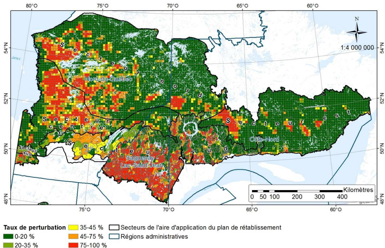
Figure 3. Taux de perturbation totale par COS ou UTR.
