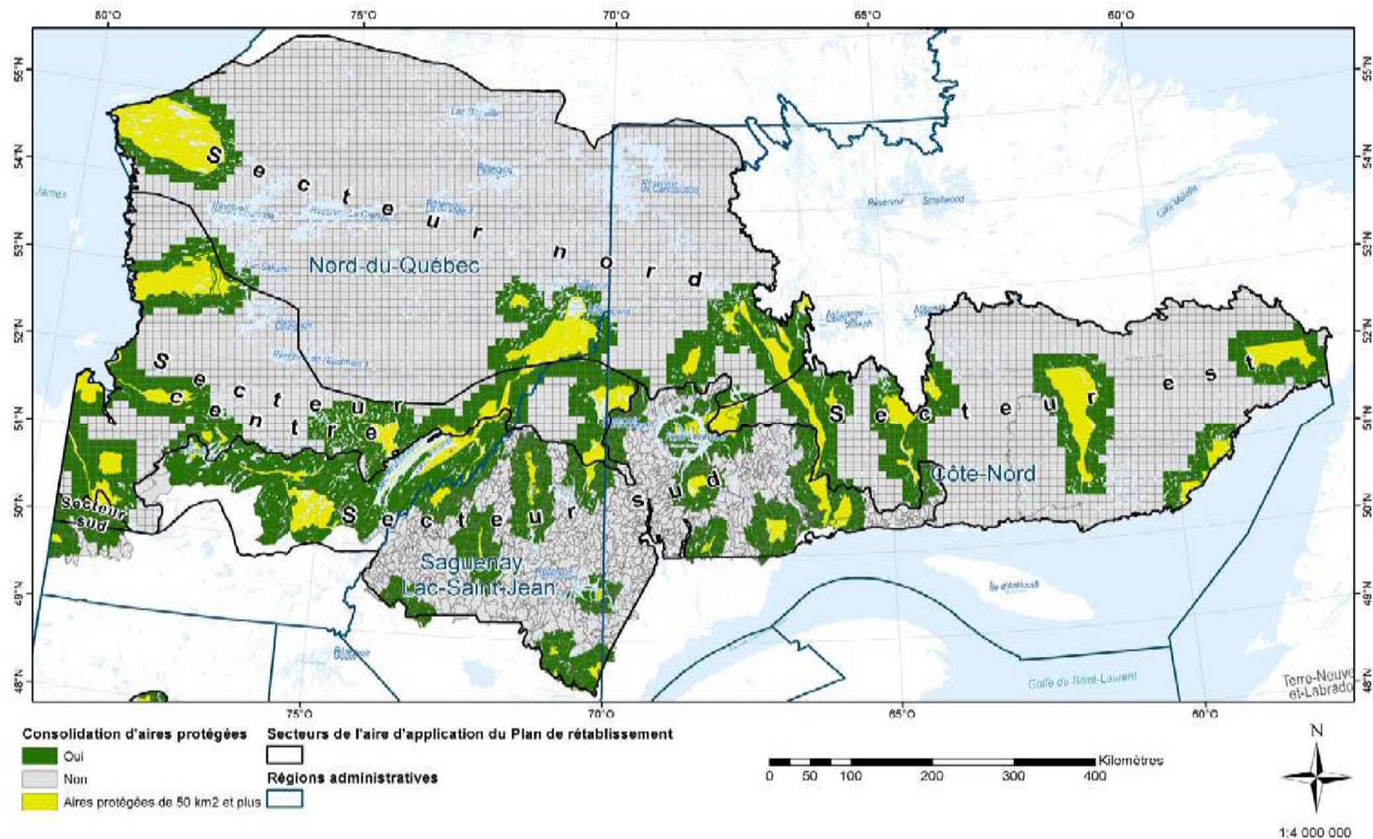
Figure A4.15. Détermination des COS ou des UTR permettant de consolider des aires protégées déjà inscrites au Registre des aires protégées.
