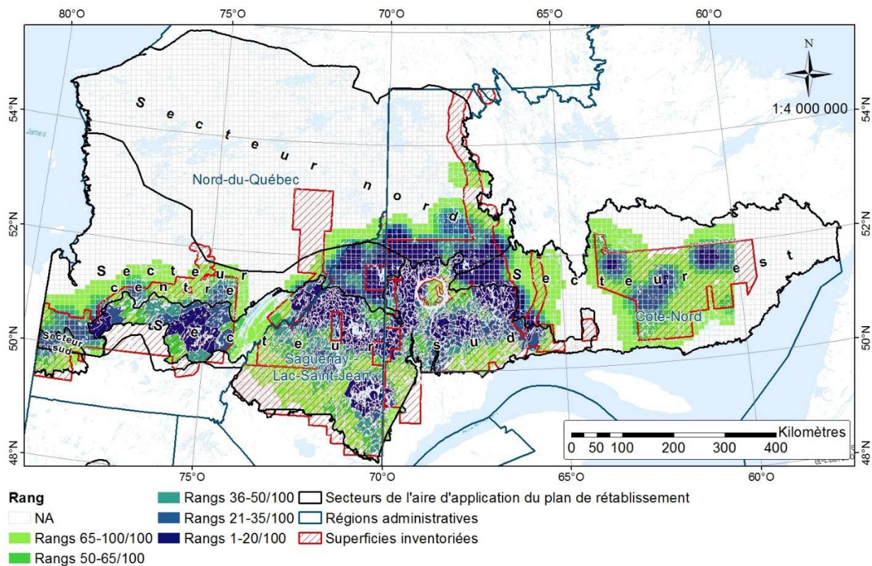
Figure 12. Variation spatiale dans les valeurs associées à l'analyse de la densité de noyaux de ravages de caribous forestiers issus des inventaires aériens, par COS ou UTR et superficies inventoriées de 1999 à 2014 ayant servi pour l'analyse de densité de noyaux.
