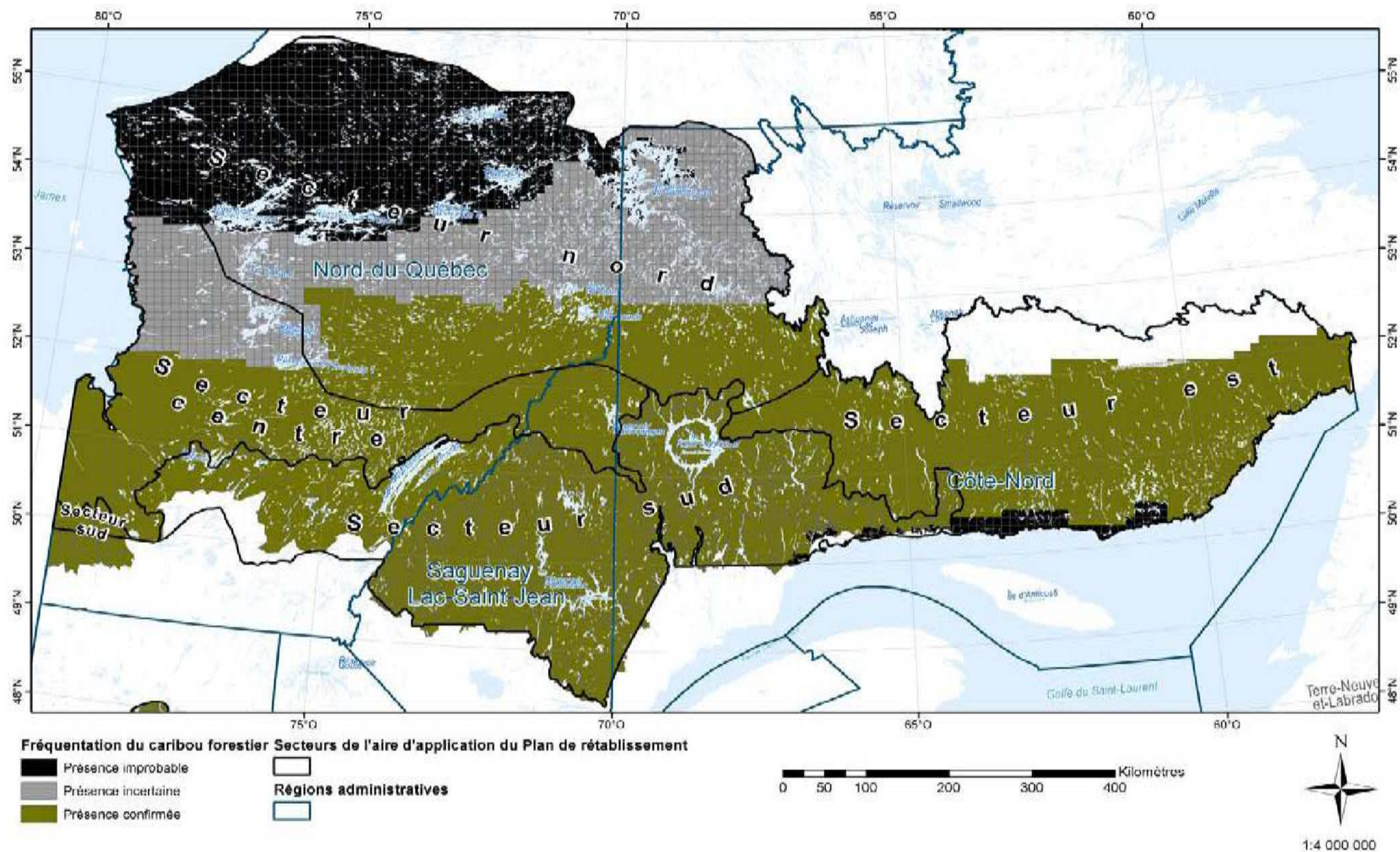
Figure A4.13. Fréquentation effective du caribou forestier d'après les observations et les connaissances pour les territoires les plus au nord et à l'est de l'aire d'application du Plan de rétablissement du caribou forestier.
