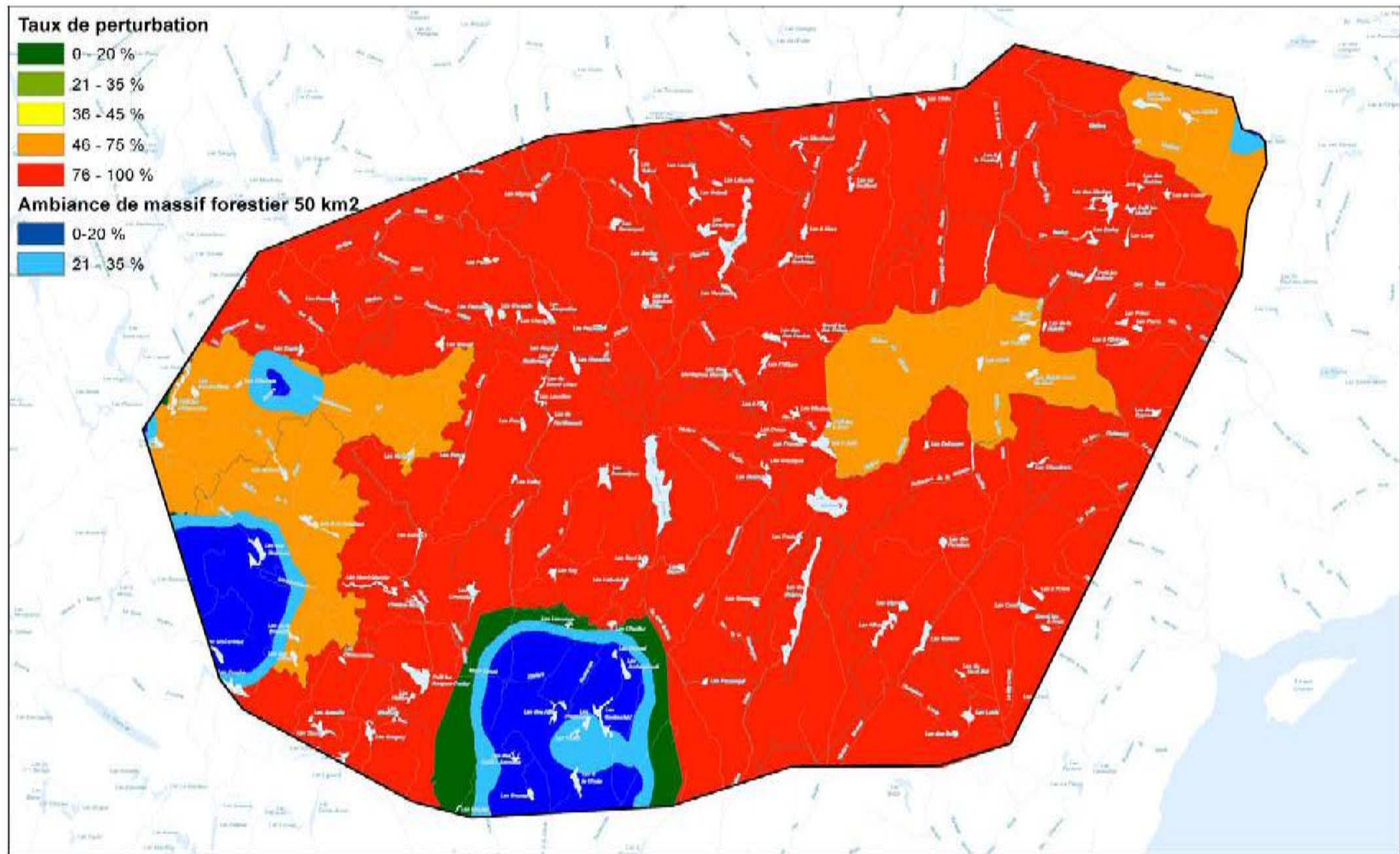
Figure A4.22. Taux de perturbation totale par COS/UTR et localisation des massifs forestiers résiduels dans le Plan d'aménagement du caribou de Charlevoix à l'aide de l'ambiance de perturbations totales à 50 km 2 .
