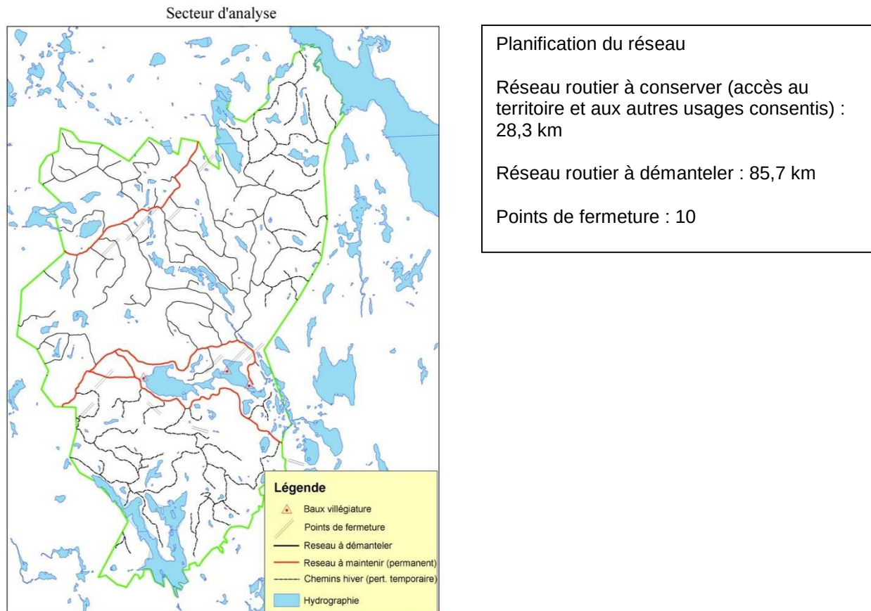
Figure A1.2. Secteur d'analyse — Analyse du réseau routier (stratégie de rationalisation du réseau routier).
