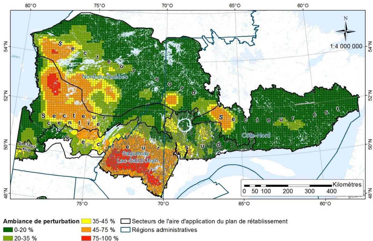
Figure 7. Ambiance de perturbations totales sur 5 000 km 2 rapportés à l'échelle du COS ou de l'UTR.
