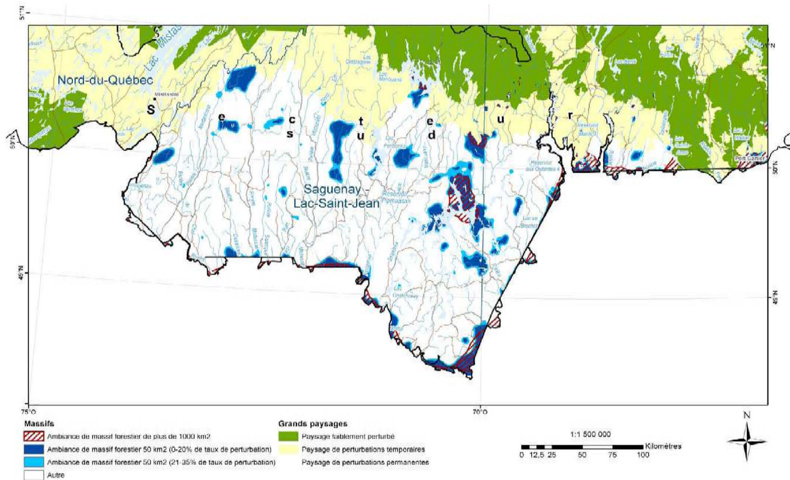
Figure A4.20. Localisation des massifs forestiers résiduels dans les paysages de perturbations permanentes et les paysages de perturbations temporaires à l'aide de l'ambiance de perturbations totales à 50 km 2 et à 1 000 km 2 .
