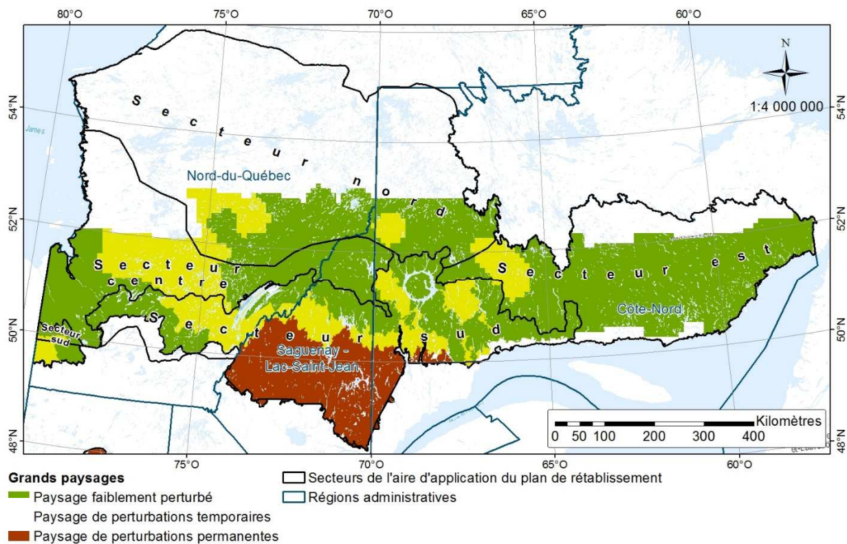
Figure 16. Délimitation des types de grands paysages dans l'aire d'application du Plan de rétablissement du caribou forestier.
