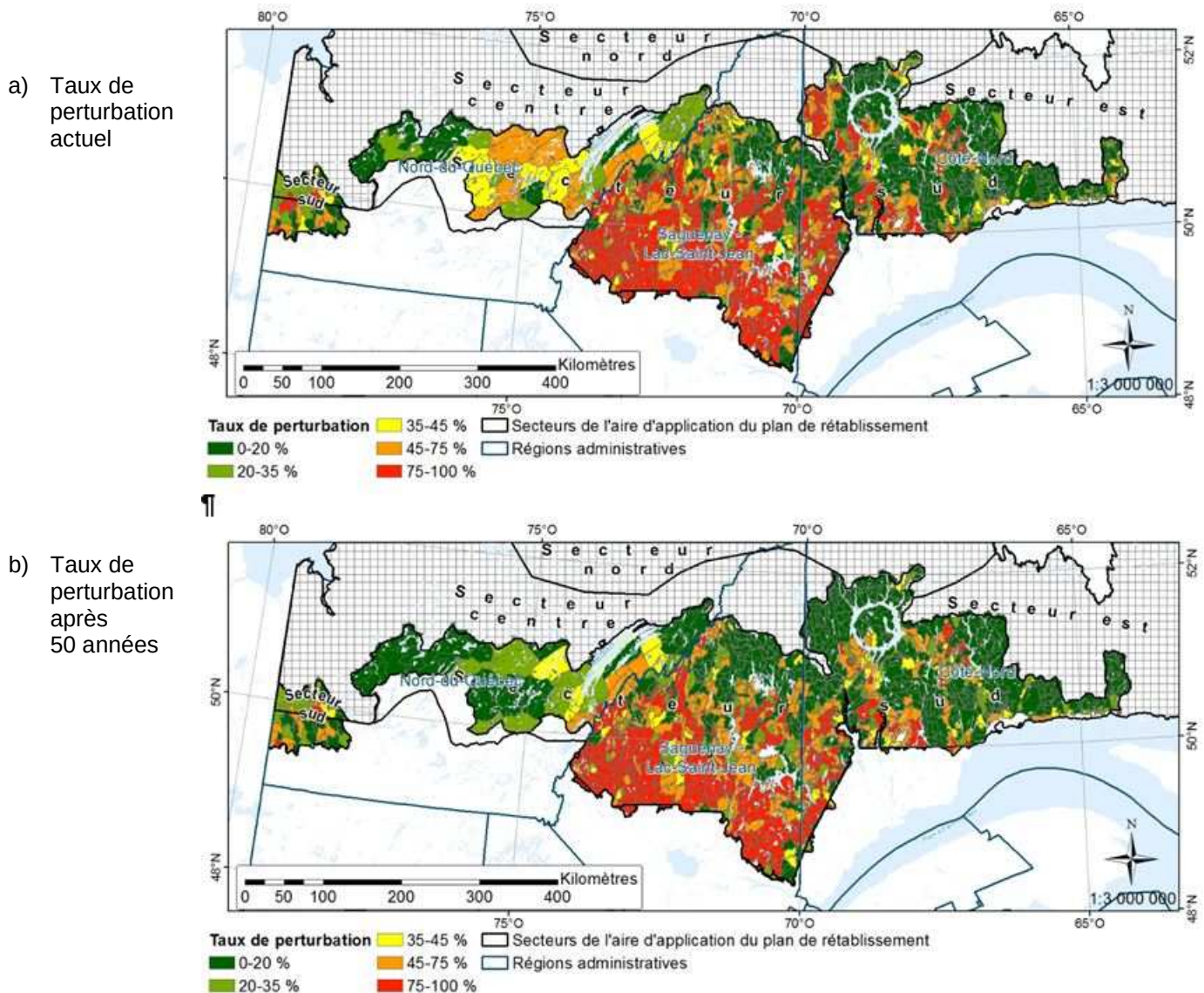
Figure 8. Évolution du taux de perturbation totale par COS ou UTR selon le modèle d'évolution naturelle théorique.
