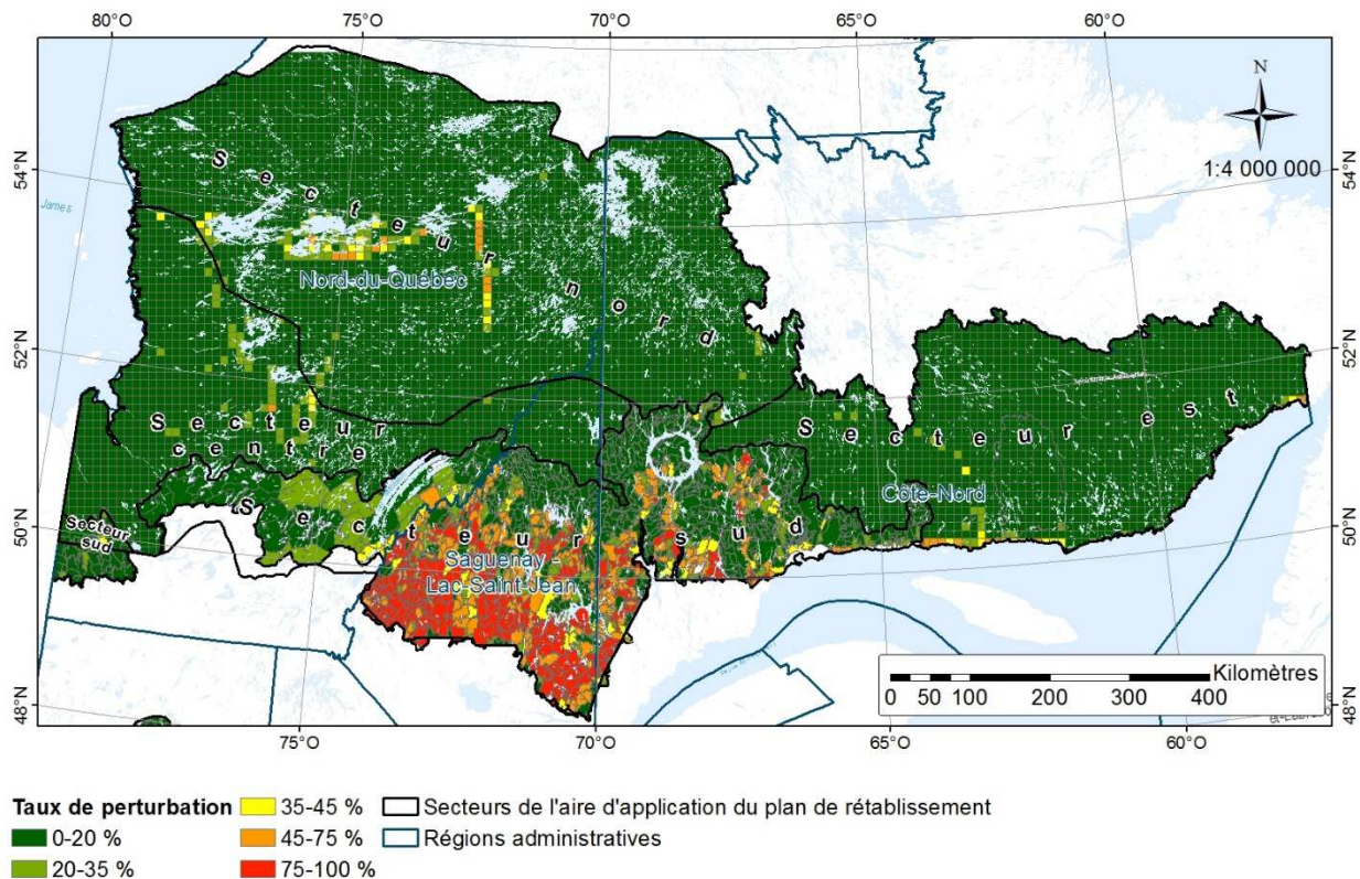
Figure 2. Taux de perturbation permanente par COS ou UTR.
