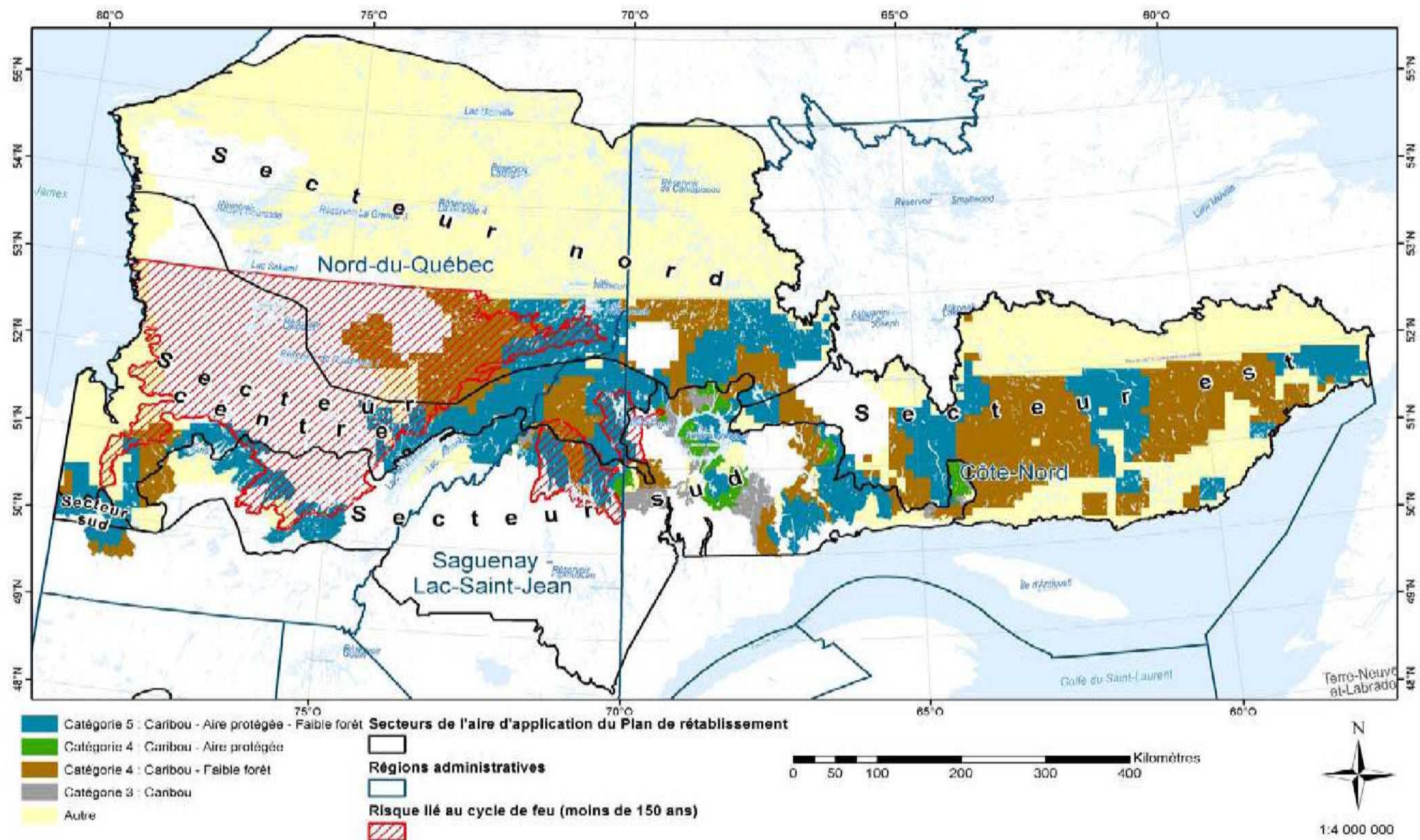
Figure A4.17. Caractérisation des paysages faiblement perturbés par leurs caractéristiques dominantes.
