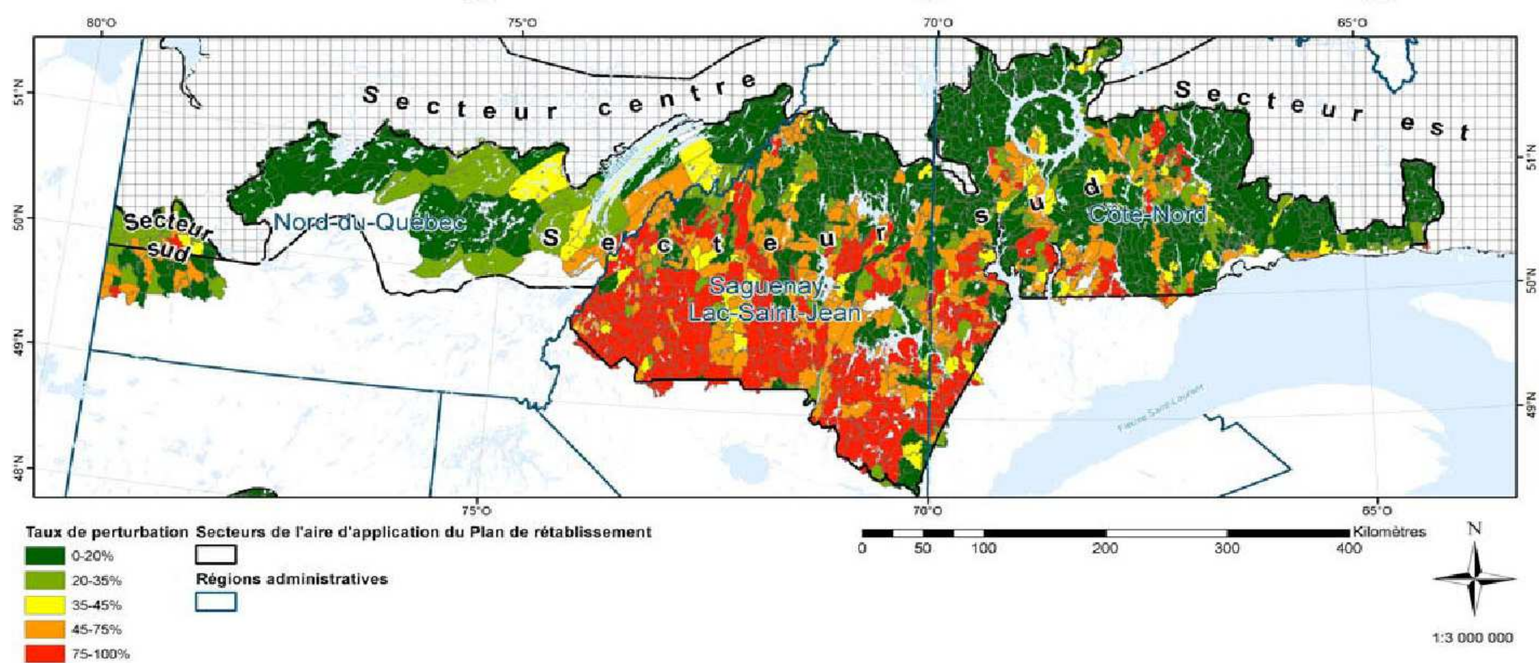
Figure A4.8. Évolution du taux de perturbation totale par COS ou UTR selon modèle d'évolution naturelle théorique.
