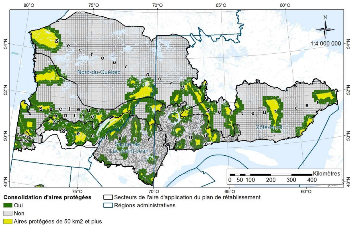
Figure 15. Détermination des COS ou des UTR permettant de consolider des aires protégées déjà inscrites au Registre des aires protégées.
