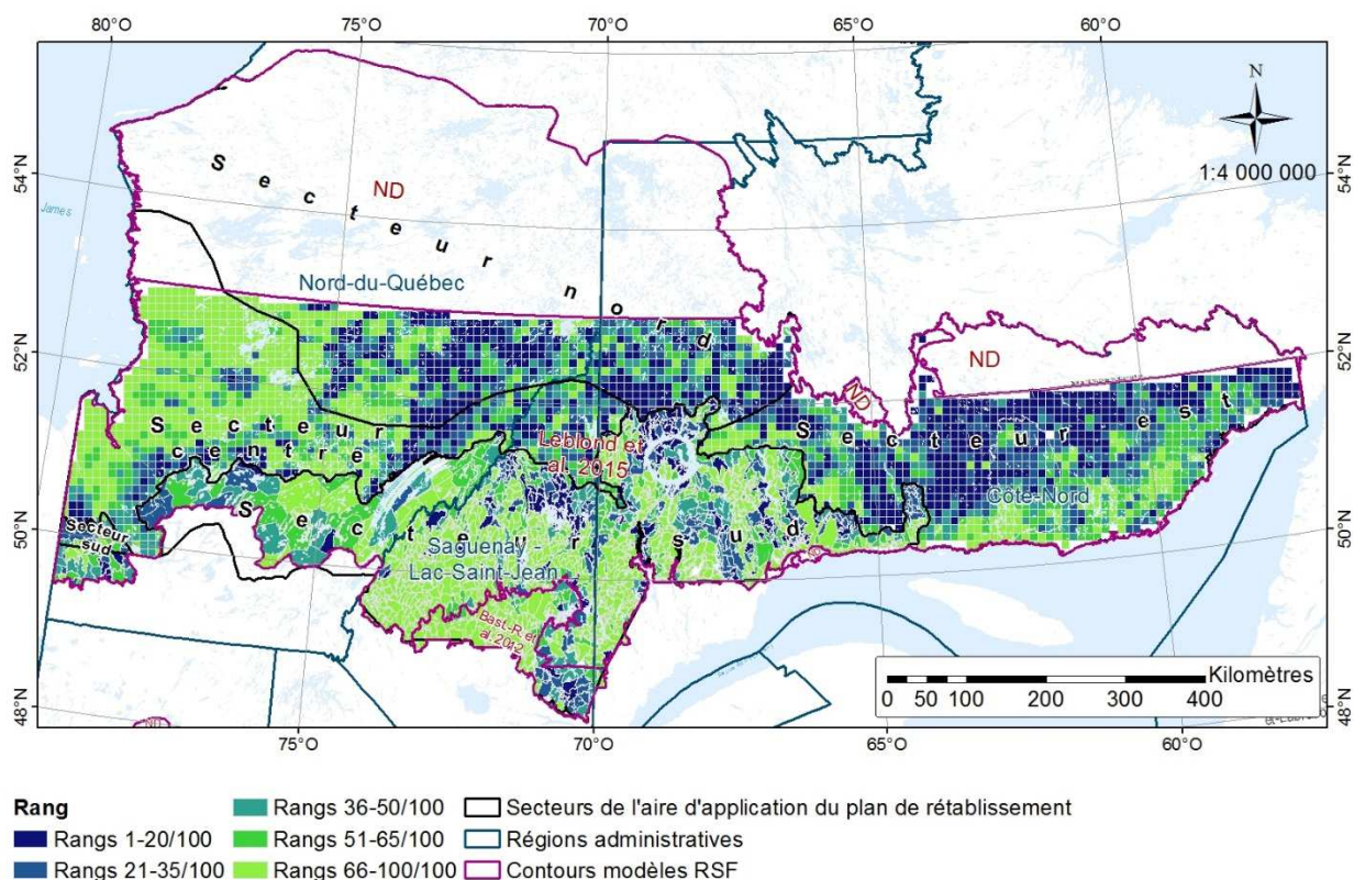
Figure 11. Indice de qualité de l'habitat pour le caribou forestier par COS ou par UTR selon les valeurs moyennes de probabilité d'occurrence relative obtenues à partir des modèles de sélection de l'habitat (Leblond et coll., 2015; Bastille-Rousseau et coll., 2012) et délimitation des superficies où ces deux modèles ont été utilisés.
