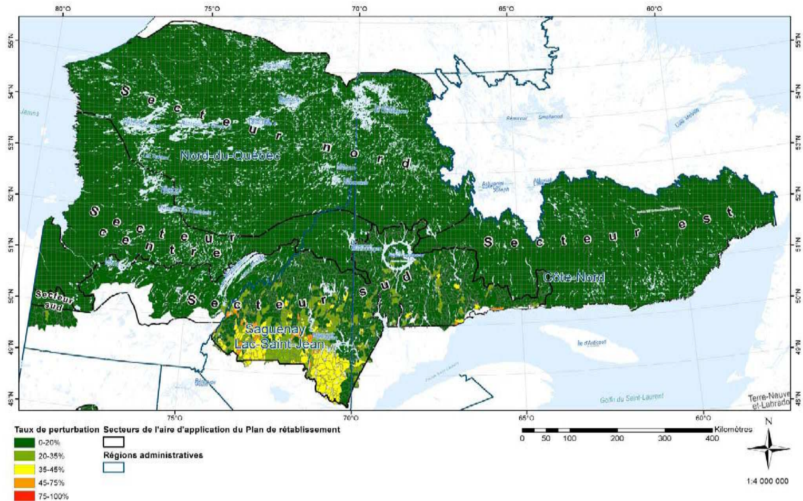
Figure A4.5. Taux de perturbation lié à l'usage d'un droit sur le territoire par COS ou UTR.
