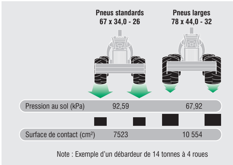
Figure 23. Impact de l'utilisation de pneus plus larges et de plus grand diamètre sur la surface de contact et sur la pression au sol pour un débardeur chargé.
