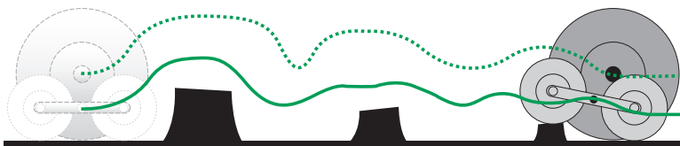
Figure 21. Comparaison du mouvement d'un essieu simple et d'un essieu tandem (Makkonen 1989 5 ).
