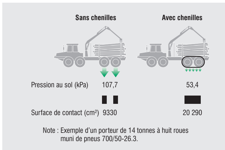
Figure 20. Impact de l'ajout de chenilles à des essieux tandems sur la surface de contact et la pression au sol d'un porteur chargé.
