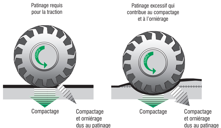
Figure 19. Poids sur la roue et patinage excessif.
