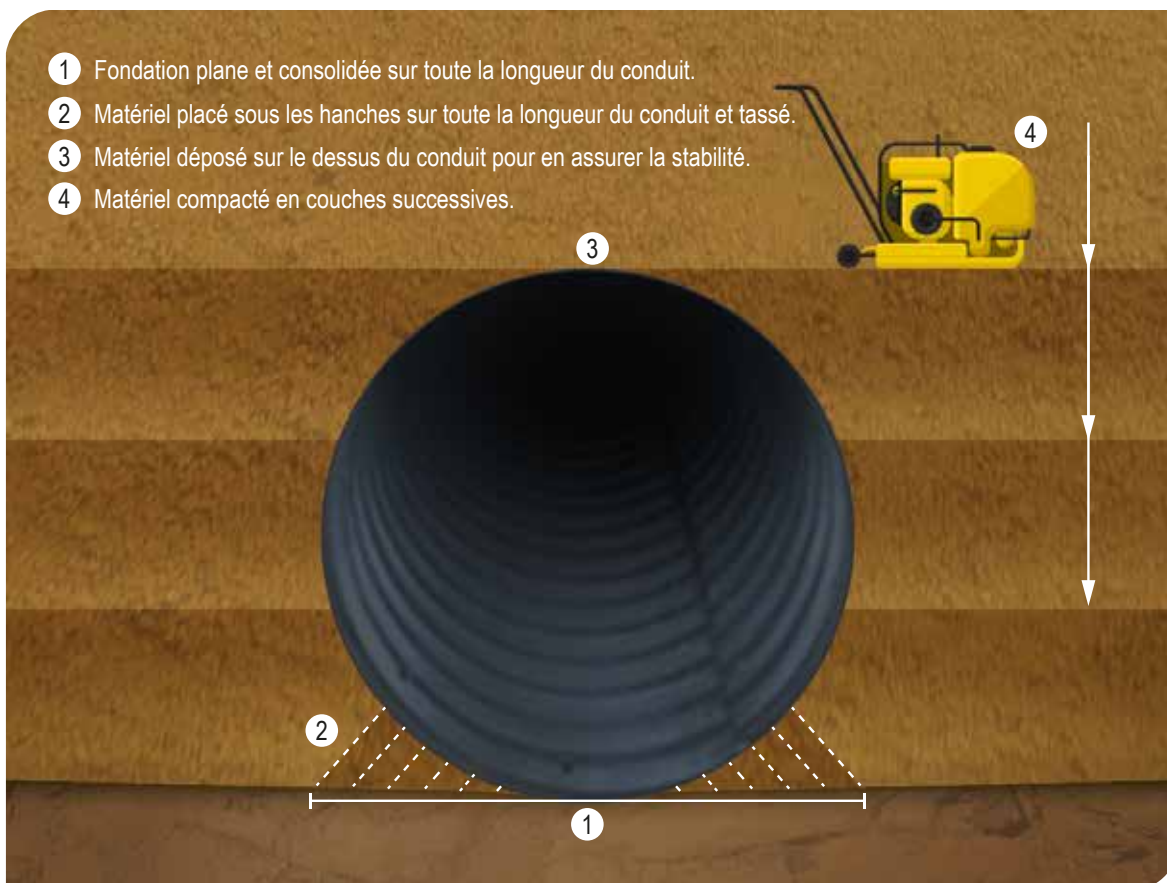
Figure 99 Remblayage d'un conduit
